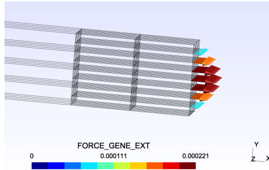
FIGURE 1 – exemple d’une résultante de répartition sinusoidale dans l’épaisseur d’une poutre (cf. 281)
