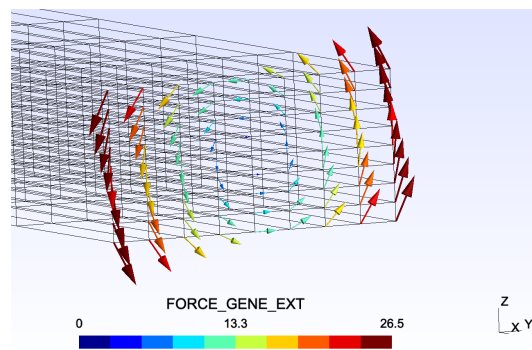
FIGURE 2 – exemple d'un moment dépendant d'une fonction nD (cf. 285)
