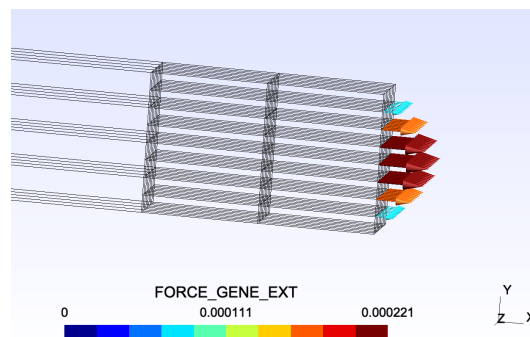
FIGURE 1 – exemple d’une résultante de répartition sinusoïdale dans l’épaisseur d’une poutre (cf. 284)
