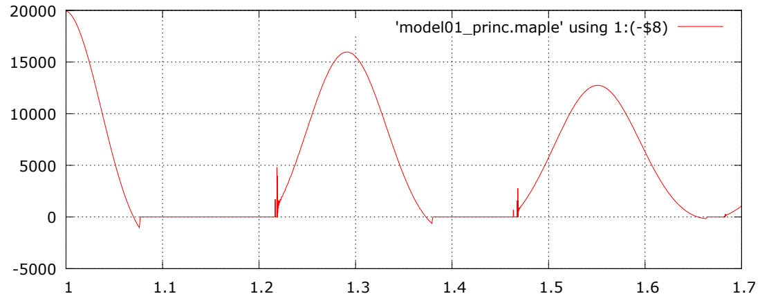
Force de réaction appui (N)
