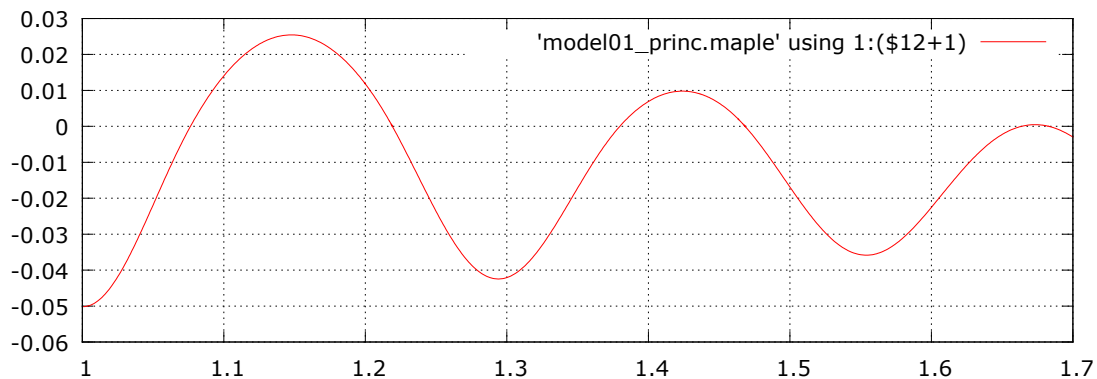
Déplacement vertical (m)
