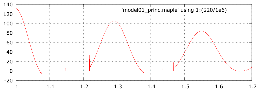
Contrainte (MPa)
