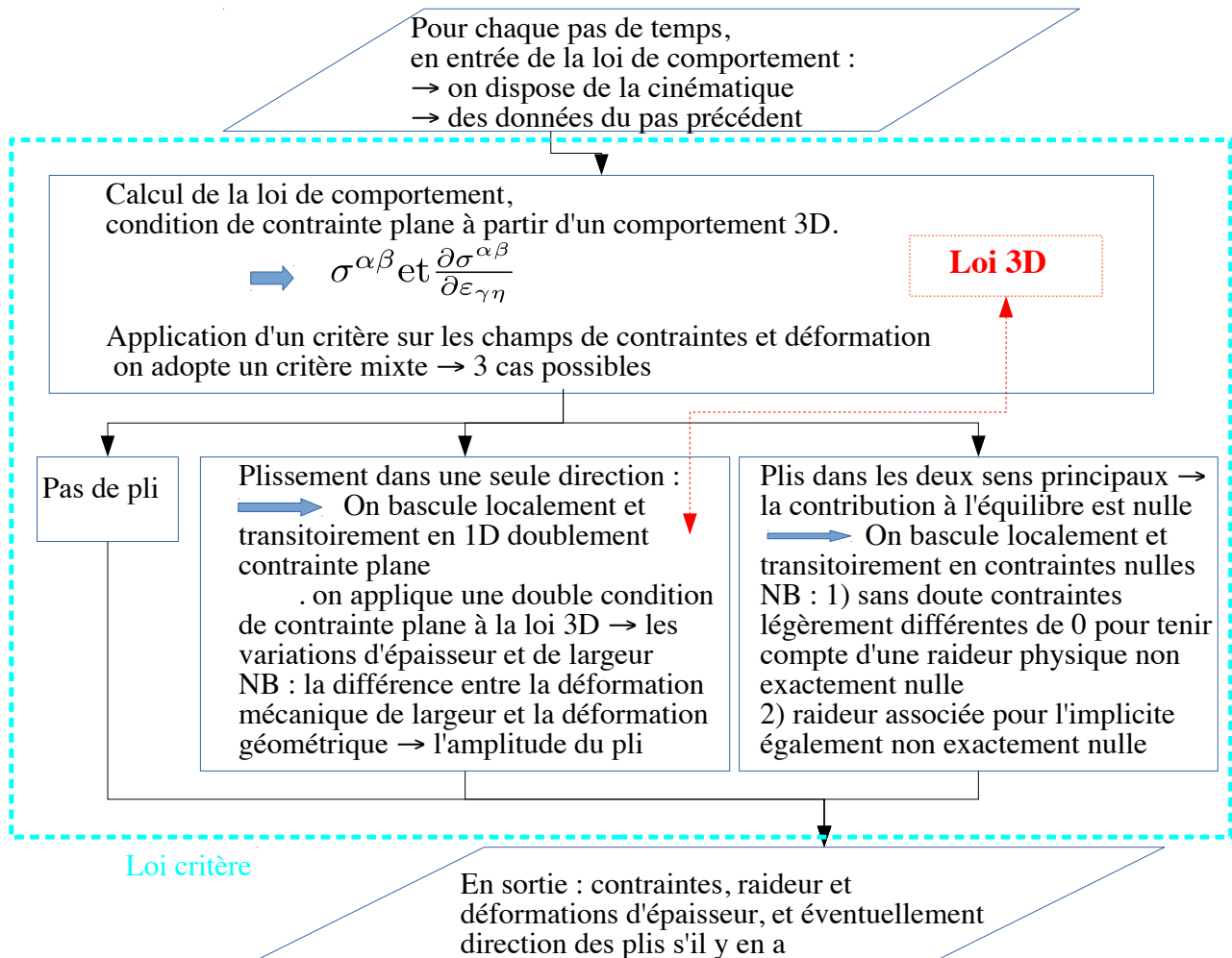
FIGURE 6 – Algorithme de traitement pour la prise en compte de plis dans le comportement mécanique macro d'une membrane
